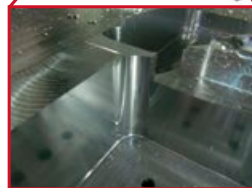
トータル(90分)加工後の刃先の損傷状態 Cutting edge after 90 minutes of milling
