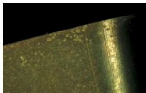
突出しが長くても欠損は無く、正常摩耗であった。
