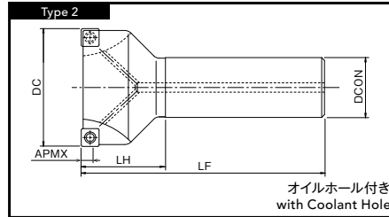
オイルホール付き with Coolant Hole
