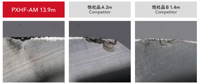
コーナR部の損耗状態 Worn state of corner R
