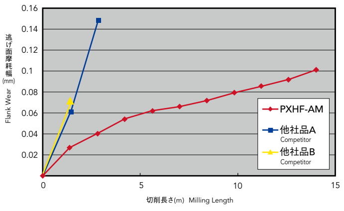
コーナR部の損耗状態 Worn state of corner R
